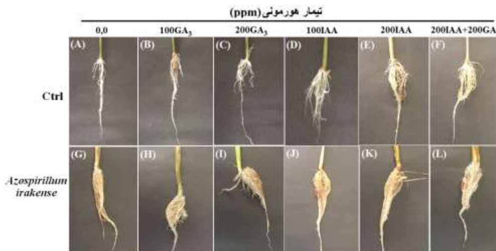
شکل ۲- ریشه گیاهچه های برنج رقم هاشمی ( O. sativa cv. hashemi ) در تیمار با غلظت های مختلف اکسین (IAA) و جیبرلین (GA3) (A-F) و یا به همراه تلقیح با ( A. irakense ) (G-L) (غلظت در شکل در تیمار هر دو هورمون مشخص شد)
