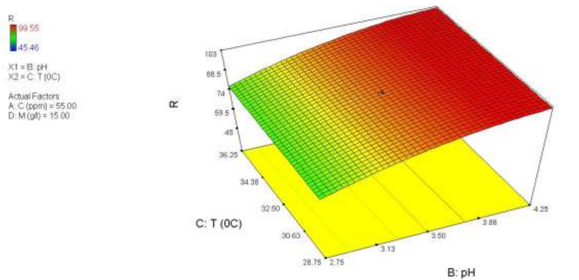
شکل ۴- سطح‌های سه‌بعدی مقدار جذب زیستی اورانیوم توسط میکروکوکوس لوتئوس. برهم‌کنش مقدار دما (°C) و pH بر میزان R. Figure 4. Three-dimensional surfaces of uranium biosorption by Micrococcus luteus . The interaction of temperature (°C) and pH on R.
