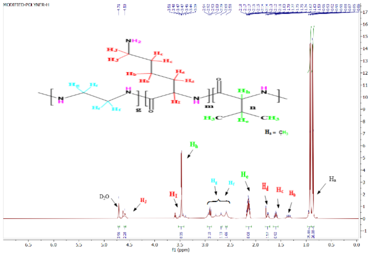
شکل ۶- طیف ^1\text{H-NMR} پلی اتیلن ایمین اصلاح شده با آمینواسید والین و لیزین.
