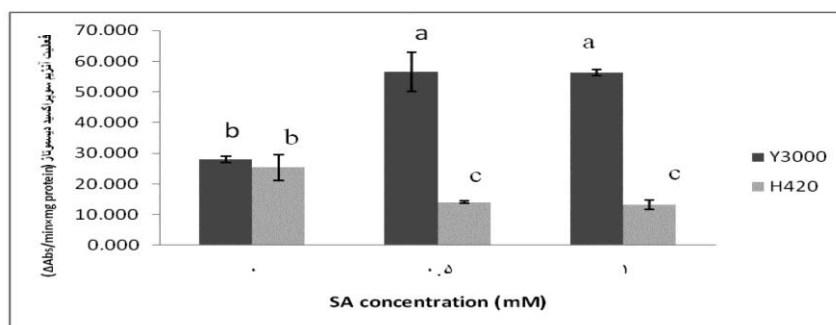
شکل ۱- فعالیت آنزیم های پراکسیداز پلی فنل اکسیداز و سوپراکسید دیسموتاز برگ در ارقام Y3000 و H420 تحت تأثیر غلظت های مختلف سالیسیلیک اسید.
